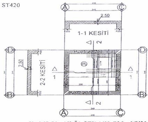
KALIP PLANI ÖLÇEK:1/50 C25 - ST420
