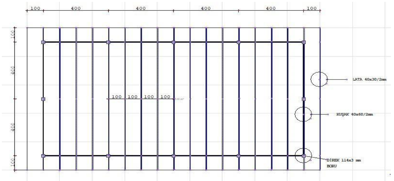
GÖLGELİK ÜST KESİT (Resim Temsilidir)
