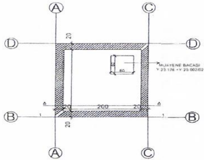
SU DEPOSU 8 m3 KULLANMA SUYU
